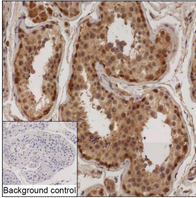
RNF212B 항체(RNF212B 마우스 근육 조직을 이용한 조직 IHC-P 분석)
