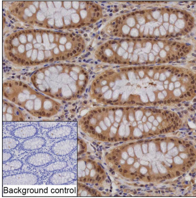
PSMA1 항체(PSMA1 마우스 단클론 항체)를 이용한 조직의 IHC-P 분석
