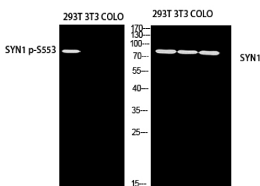
SYN1 抗体を用いた 293T 3T3 COLO のウェスタンブロット解析。抗体は 1:1000 に希釈した。二次抗体は 1:20000 に希釈した。
